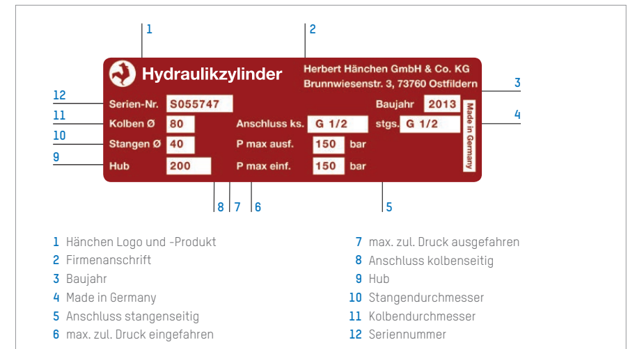
Abbildung 1: Beispiel Typenschild Hydraulikzylinder
