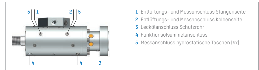
Abbildung 7: Entlüftungs- und Messanschlüsse Zylinder Dichtungssystem Servobear®
