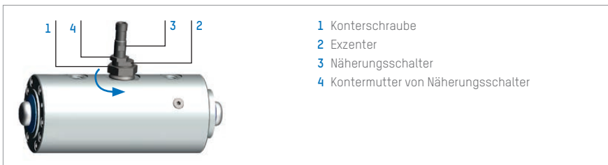
Abbildung 13: Näherungsschalter auf entriegelt stellen
