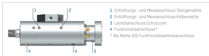
Abbildung 6: Entlüftungs- und Messanschlüsse Zylinder Dichtungssystem Servofloat®
