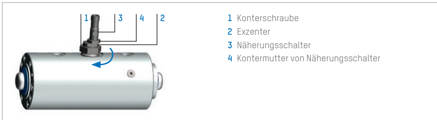
Abbildung 12: Näherungsschalter auf verriegelt stellen
