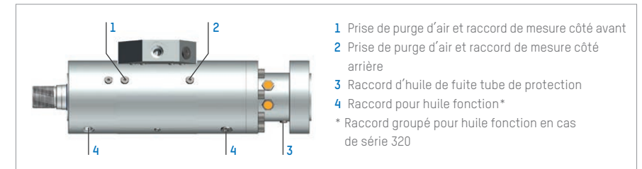
Illustration 6 : Prises de purge d'air et raccords de mesure du système de joints du vérin Servofloat®
