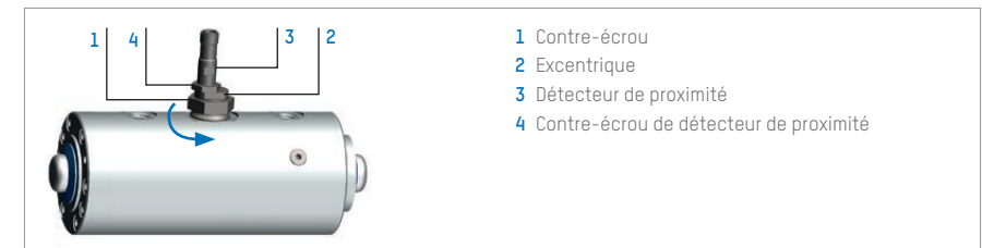
Illustration 13 : Régler le détecteur de proximité sur déverrouillé
