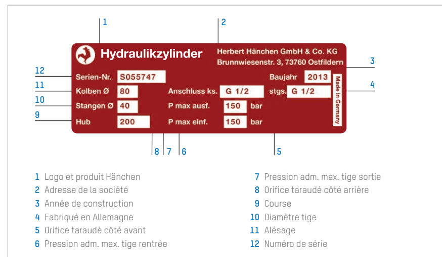
Illustration 1 : Par exemple plaque d'identification du vérin hydraulique
