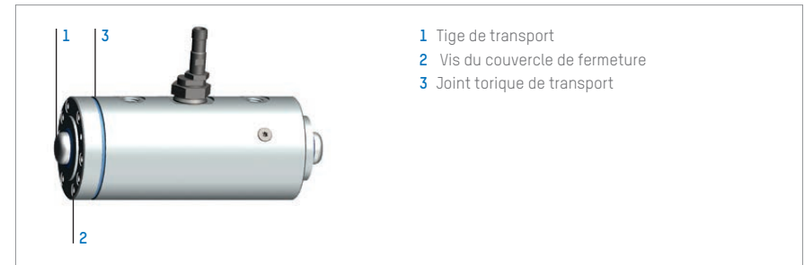
Illustration 14 : Montage du bloqueur de tige Ratio-Clamp®
