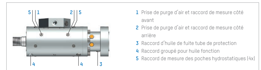
Illustration 7 : Prises de purge d'air et raccords de mesure du système de joints du vérin Servobear®
